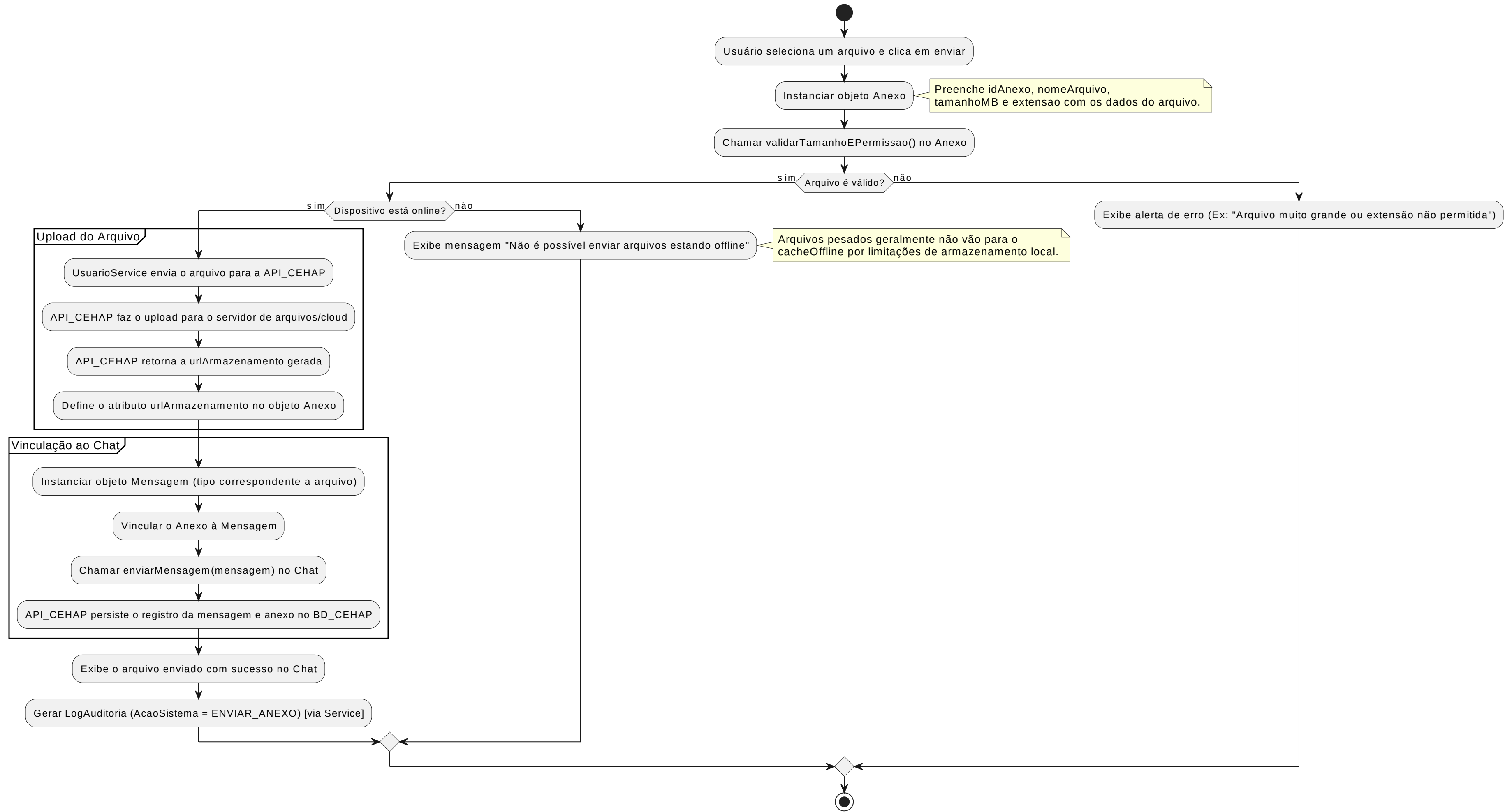
Diagrama de Atividade - Método enviarArquivo()
